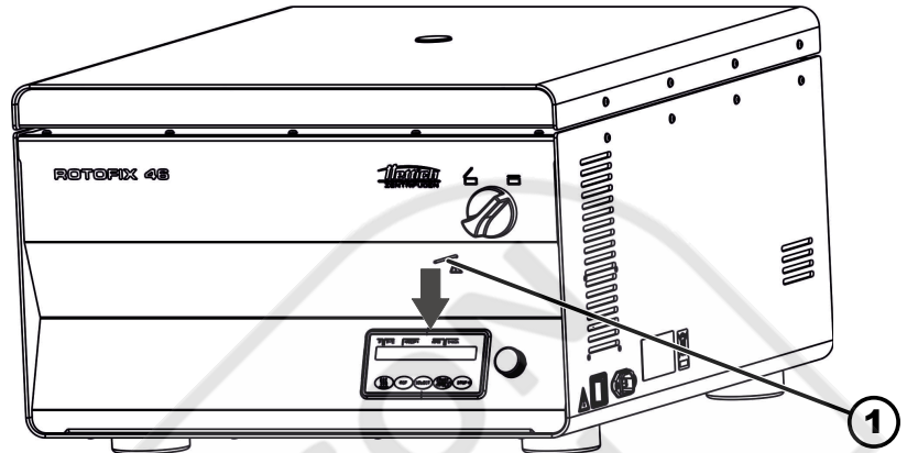
Abb. 17: Notentriegelung
