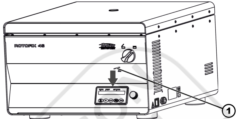
Fig. 17 : Déverrouillage d'urgence
